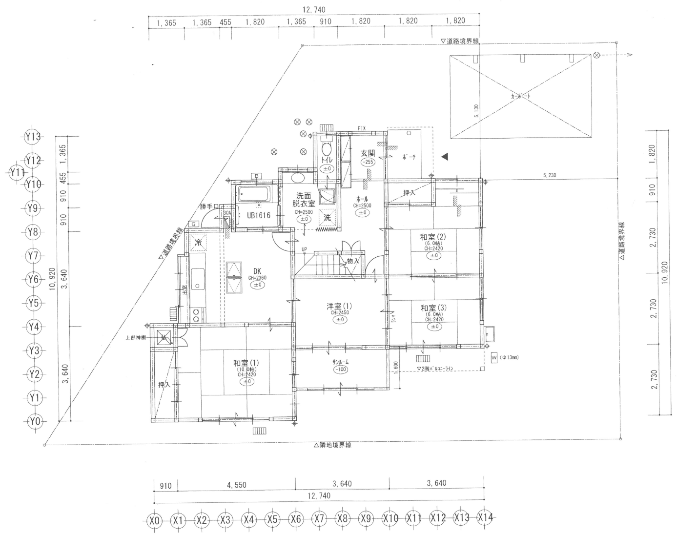
1階平面図
